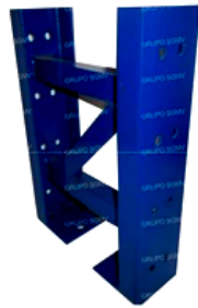
Marco de racks calibre 12, 14 y 16, paso 5.
